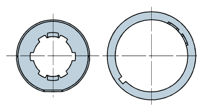
515.25003 Scheibe 50x(1,3-1,5) Rad + Ausgleichskranz
