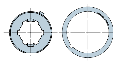
515.25004 Scheibe mit Verrippung und Innenlasche 47, Rad + Ausgleichskranz
