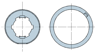
515.25002 Scheibe 50x1,5 Rad + Ringkranz
